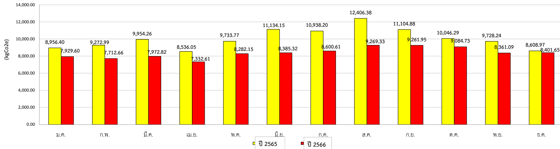
เปรียบเทียบปริมาณก๊าซเรือนกระจกเดือนมกราคม - ธันวาคม ปี พ.ศ.2565 และ ปี พ.ศ. 2566
