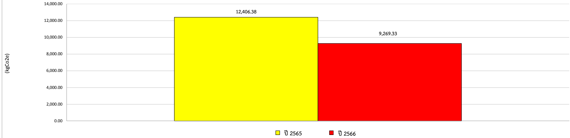
เปรียบเทียบปริมาณก๊าซเรือนกระจกเดือนสิงหาคม ปี พ.ศ.2565 และ ปี พ.ศ. 2566
