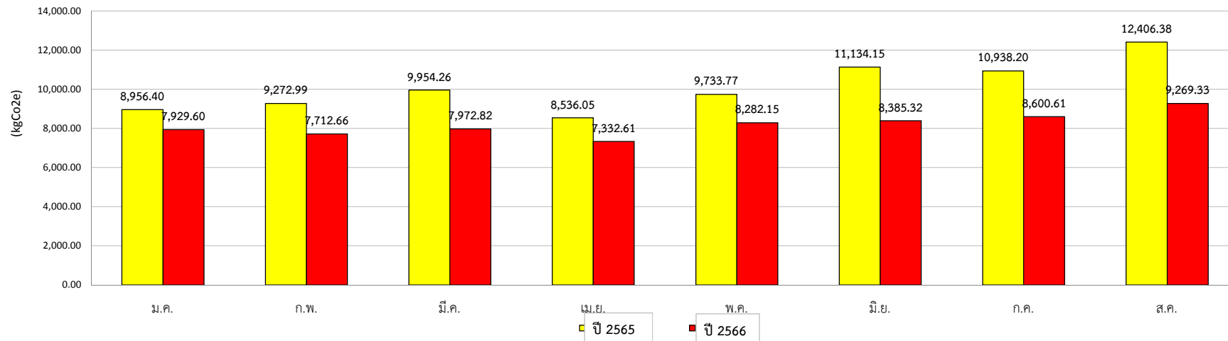
เปรียบเทียบปริมาณก๊าซเรือนกระจกเดือนมกราคม - สิงหาคม ปี พ.ศ.2565 และ ปี พ.ศ. 2566
