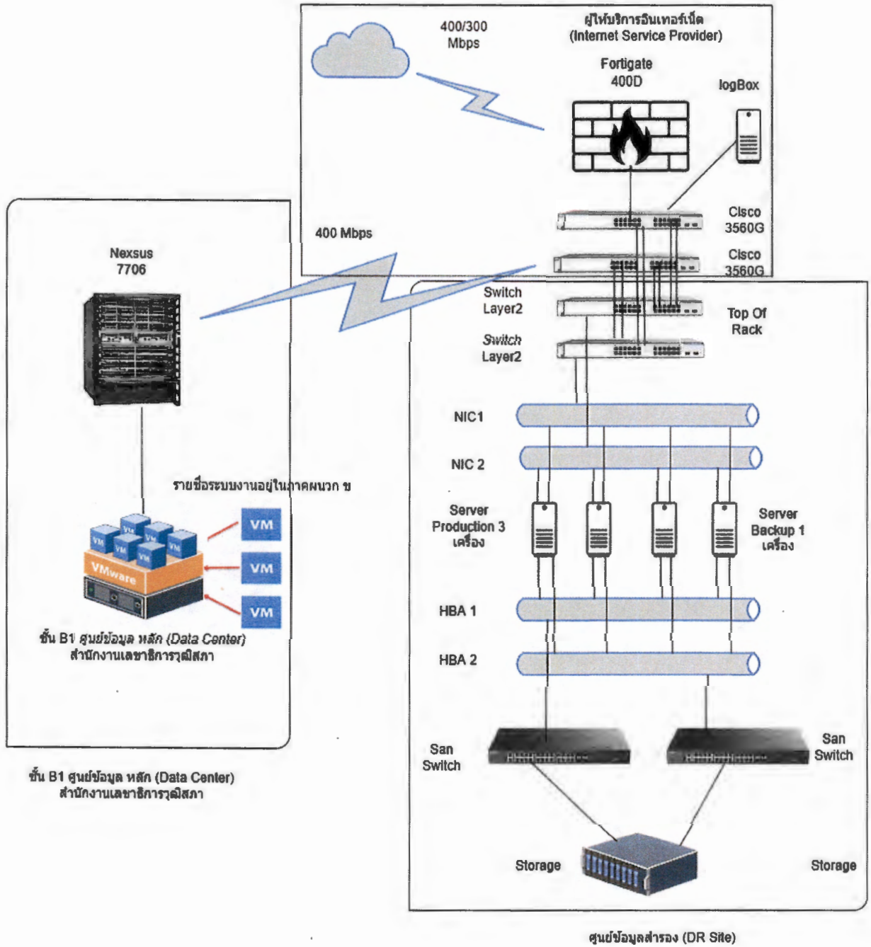
Diagram โครงการจัดซื้อครุภัณฑ์อุปกรณ์ศูนย์ข้อมูลสำรอง (DR Site) สำนักงานเลขาธิการวุฒิสภา
